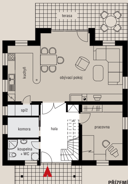
PŘÍZEMÍ
